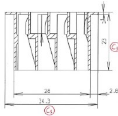
COUPE A-A
